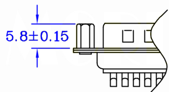
前鉚型(不通孔)
