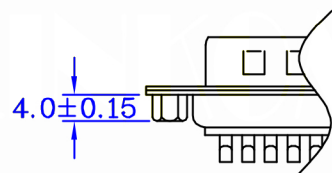
後鉚型(通孔)
