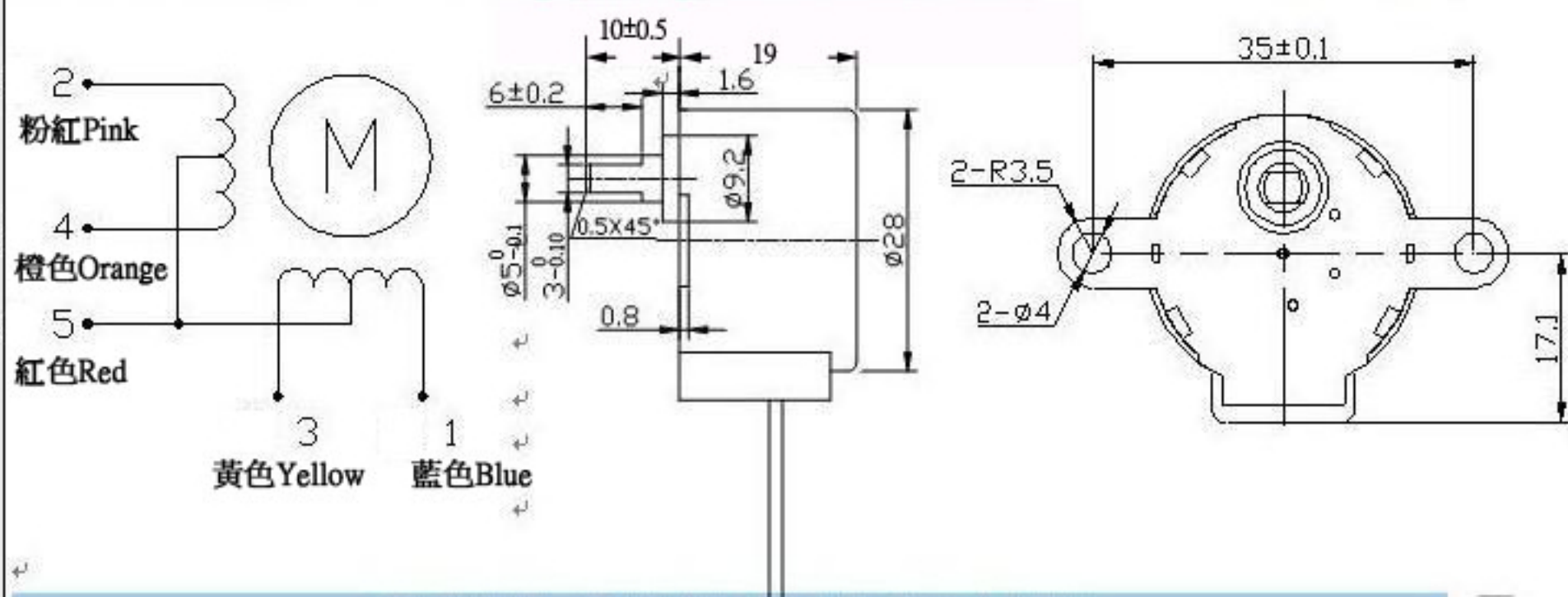
接線示意圖: Wiring diagram
