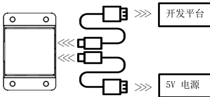
图 4 YDLIDAR S4 辅助供电
