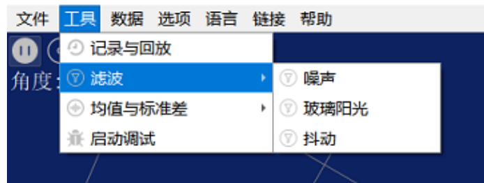
图 17 滤波设置
