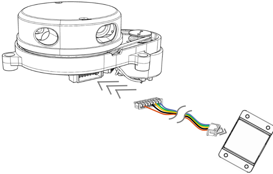
图 2 YDLIDAR S4 设备连接 STEP 1
