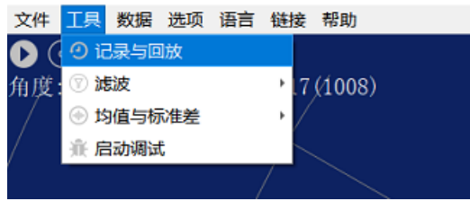
图 14 记录与回放
