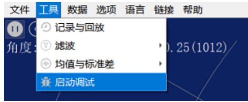
图 16 启动调试
