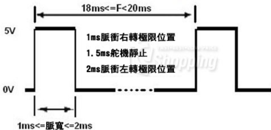
舵機信號控制圖
